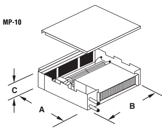
MP-10 RACCORD DU CONDUIT D'ARRIVÉE D'AIR 12 X 4 RACCORD DU CONDUIT DE SORTIE D'AIR 3 1/4 X 10 DIMENSIONS DU FILTRE 12 X 3 1/2 X 1/2, RÉUTILISABLE
