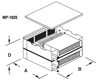
MP-1020 RACCORD DU CONDUIT D'ARRIVÉE D'AIR 12 X 8 RACCORD DU CONDUIT DE SORTIE D'AIR 7 1/4 X 10 DIMENSIONS DU FILTRE 12 X 7 1/2 X 1/2, RÉUTILISABLE
